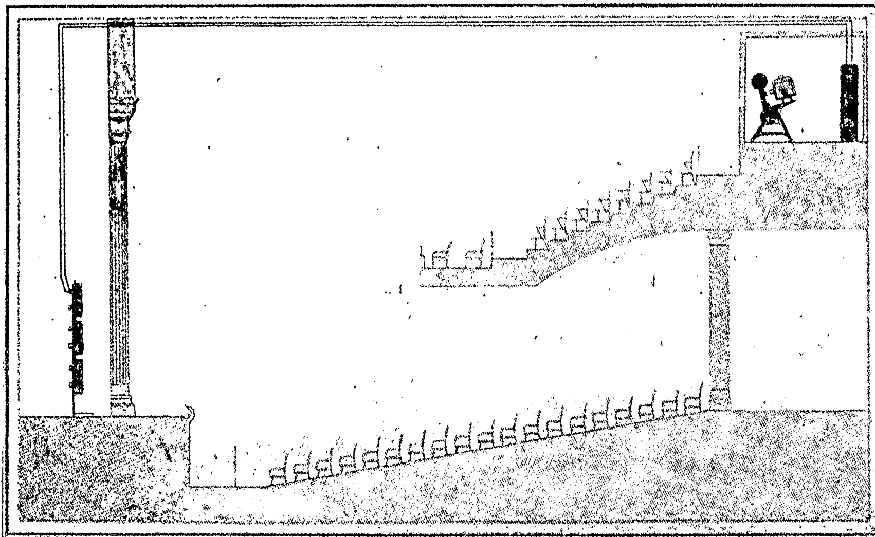
Схема кино-театра с оборудованием для звуковых фильм. Справа наверху аппаратная камера с проектором и усилителем, откуда провода ведут к громкоговорителям установленным на сцене за экраном. (На рисунке слева).
